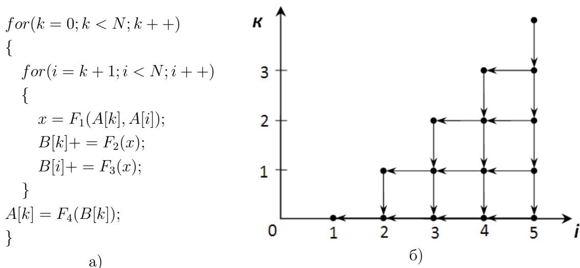
Рис. 4. Схема информационных зависимостей алгоритма формирования режущей части инструмента
